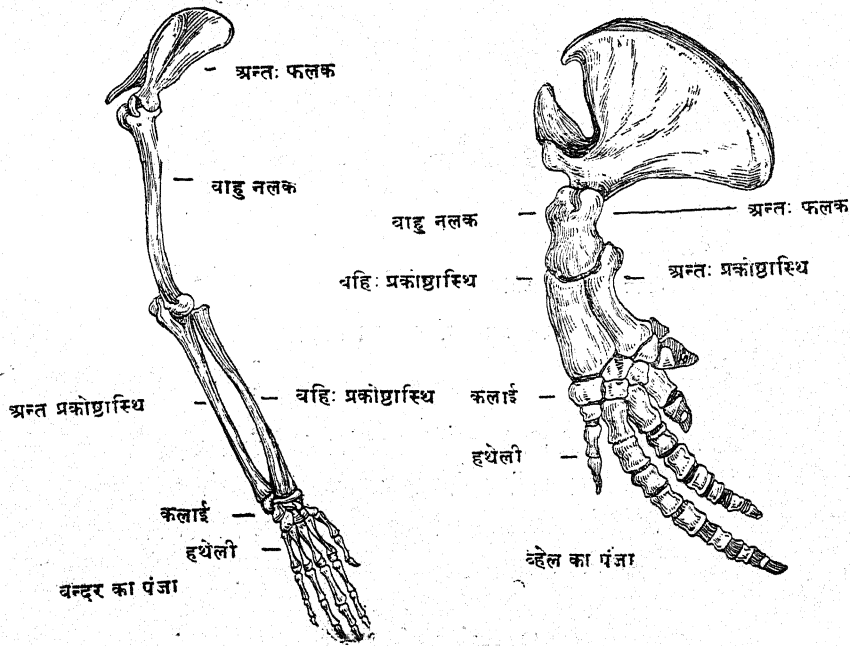
चित्र ७७—पंजे का क्रमिक विकास
